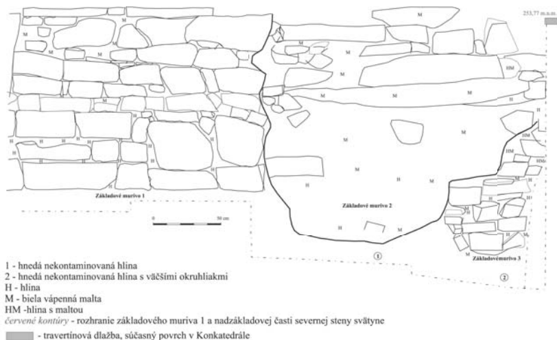
Konkatedrála sv. Mikuláša v Prešove. Grafická dokumentácia základových murív 1-3 severnej steny svätyně. Kresba: M. Čurný.
